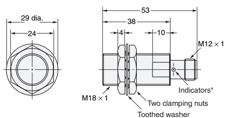
Diagram 24 E2E-X7D□-M1(G)/E2E-X5E□-M1/X5F□-M1 E2E-X5Y□-M1
