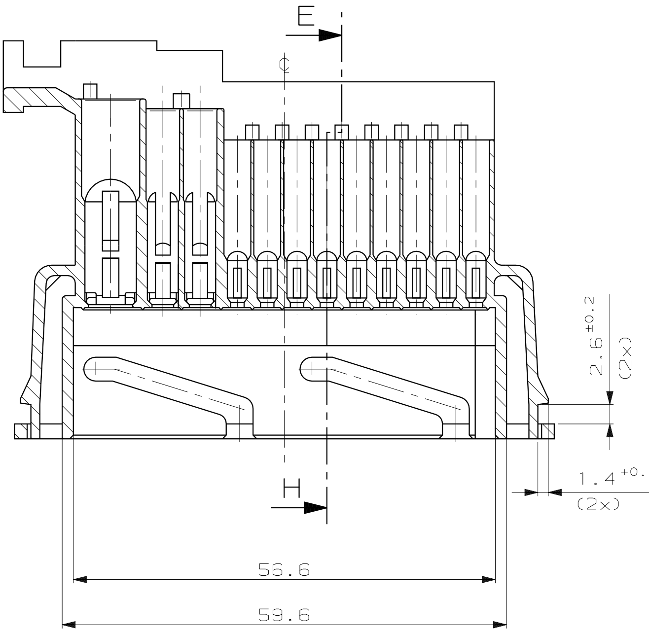
Schnitt SECTION J-K
