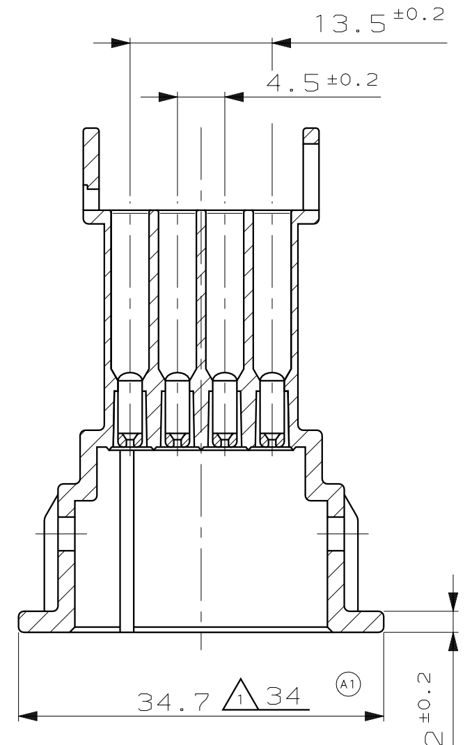
Schnitt SECTION E-H
