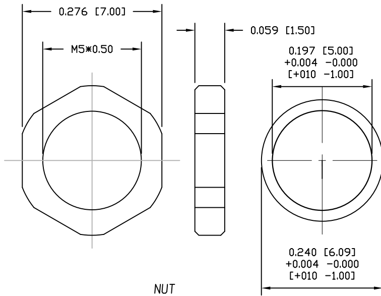
NUT
