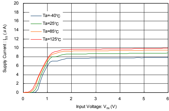
XC6130 ( V_{DF(T)}=1.6V )
