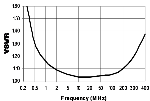
Output VSWR
