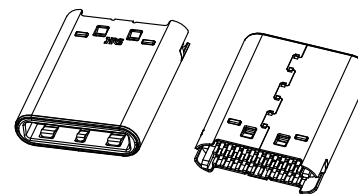
ISO-VIEW(N/S)
