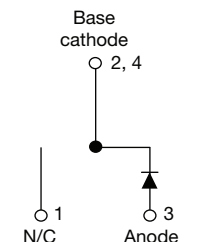
VS-ETU1506SHM3
