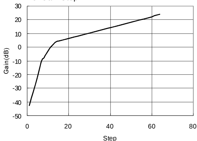
18. Gain Step
