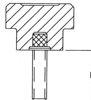
THREADED STUD
