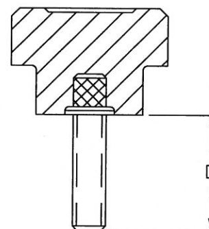
THREADED STUD
