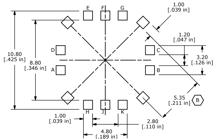
P.C.B. LAYOUT
