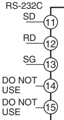
E53-CN01N2 Communications (RS-232C)
