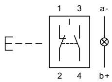
Wiring diagram 24
