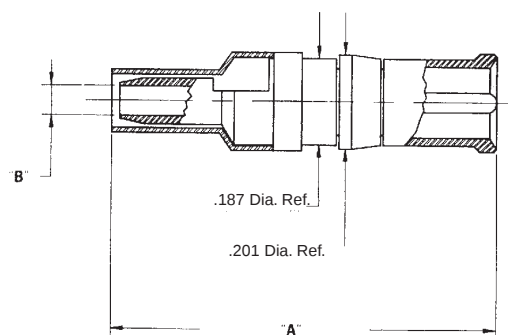
Receptacle
