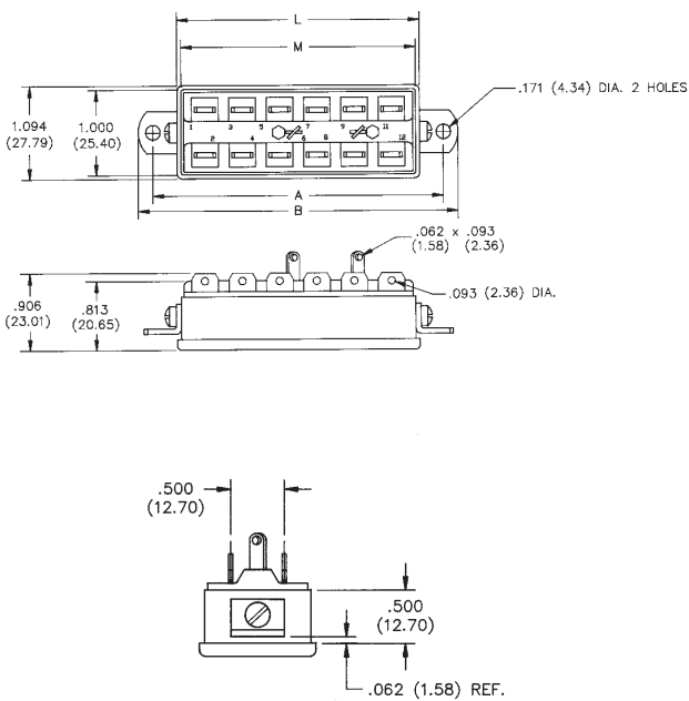
Socket
