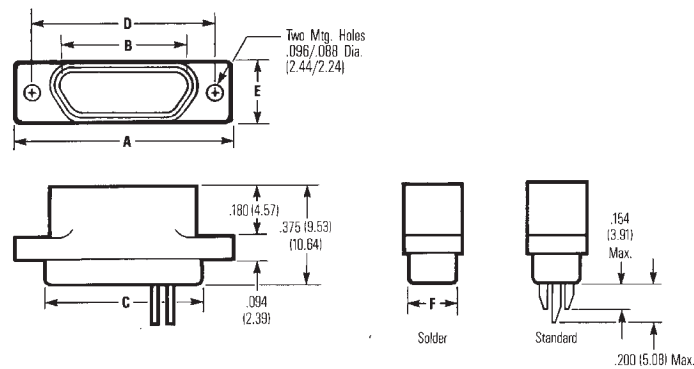
Socket
