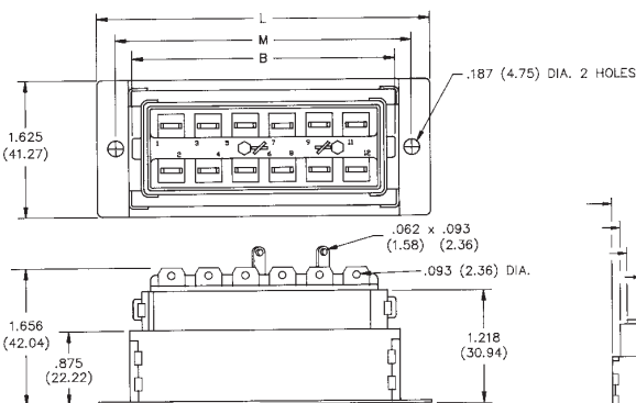
Socket
