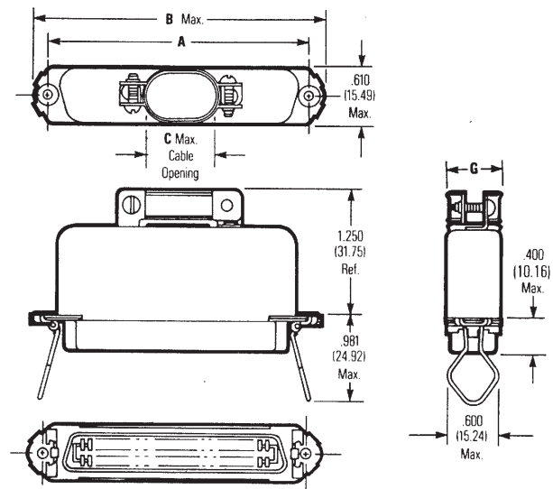
Socket
