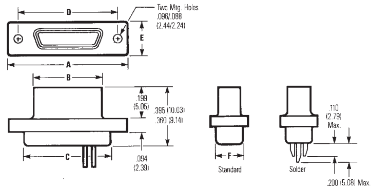
Socket
