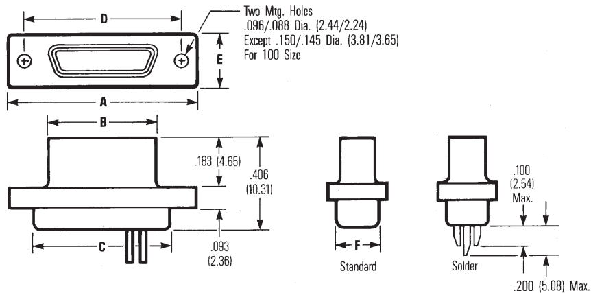
Socket
