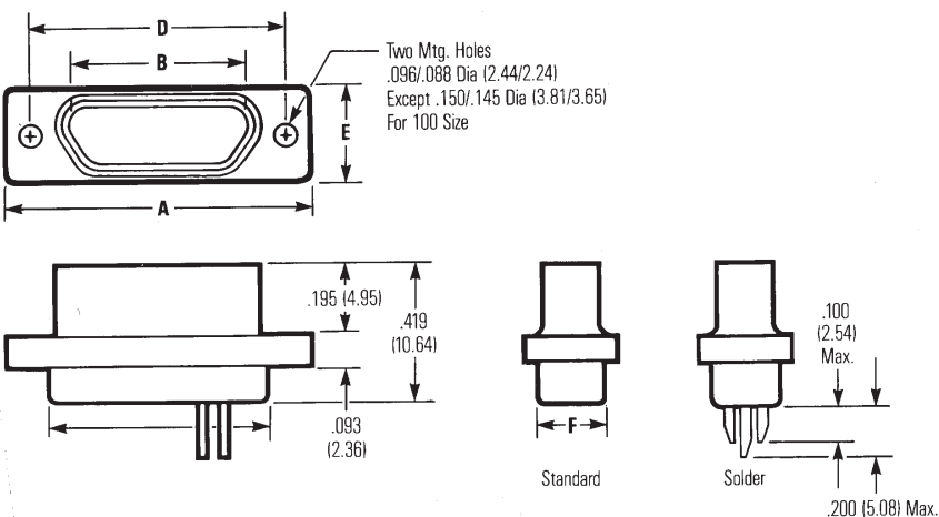
Socket
