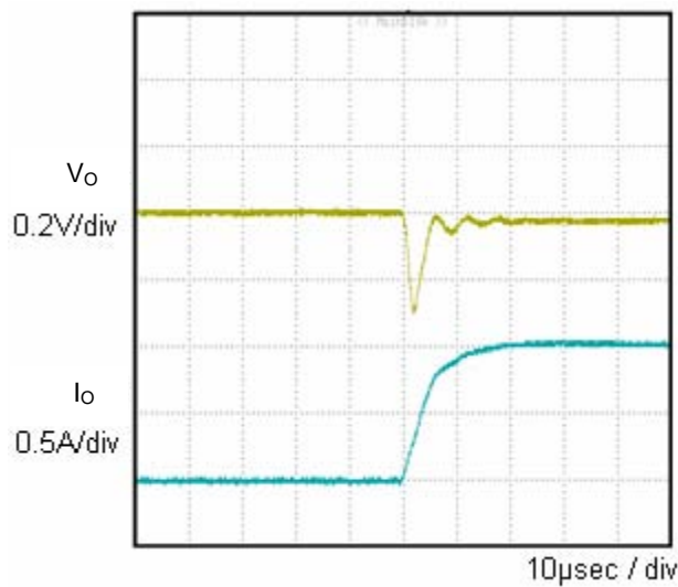
Fig.3 Transient Response(0→1.0A) Co=1.0μF
