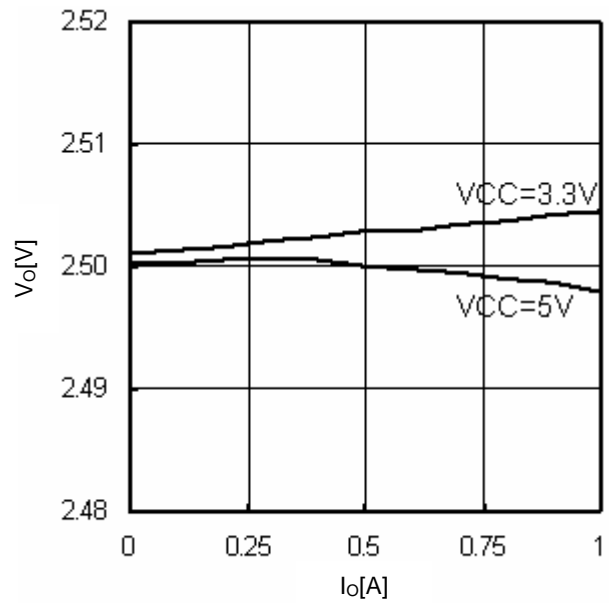
Fig.18 I_o-V_o ( V_o=2.5V )
