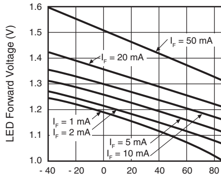
ih1546aef_01 T_A - Ambient Temperature ( ^{\circ}\text{C} )
