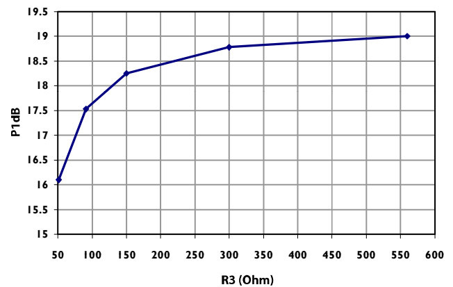
P1dB
