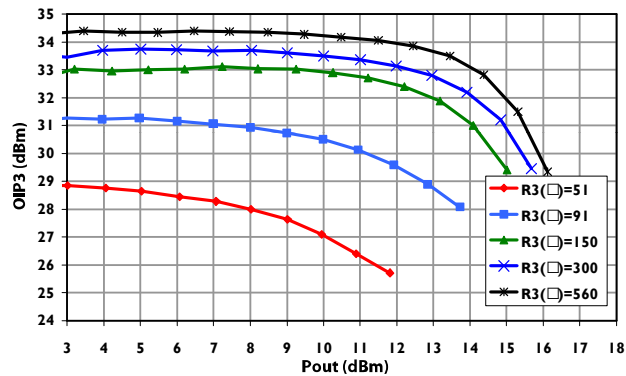
OIP3
