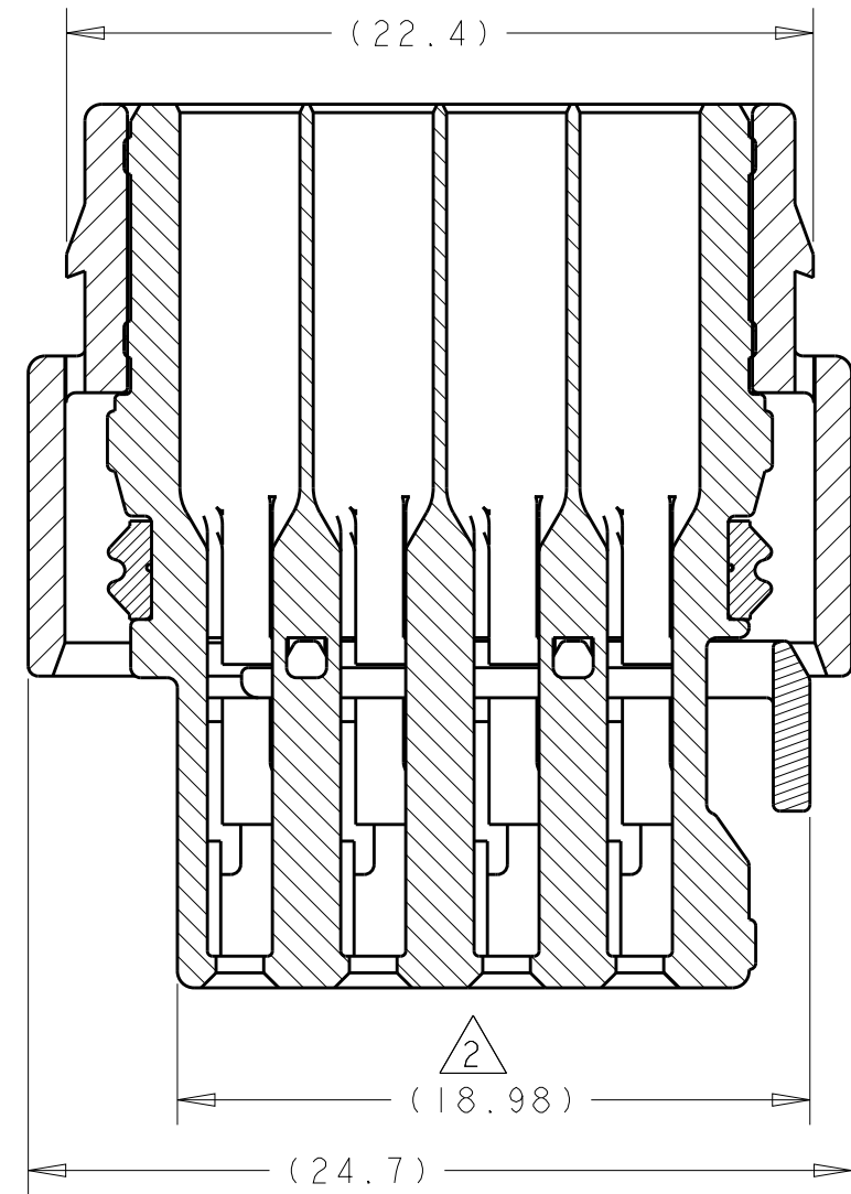
SECTION A-A
