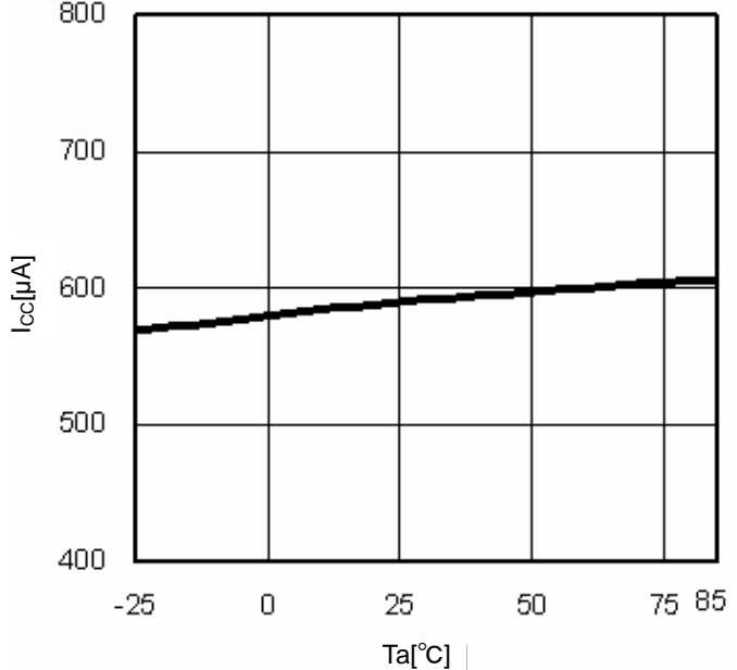
Fig.9 T_a-I_{cc}
