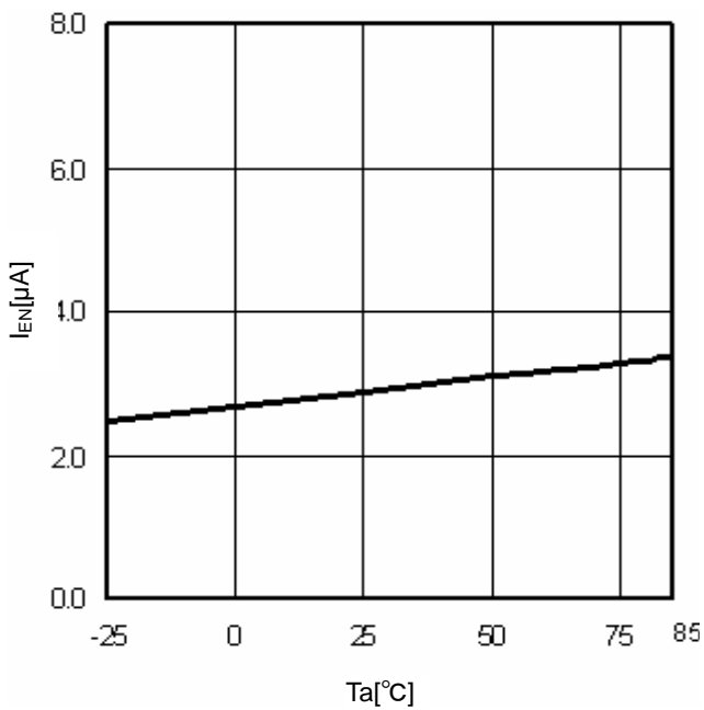
Fig.11 T_a - I_{EN}
