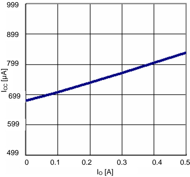
Fig.19 I_o - I_{cc}
