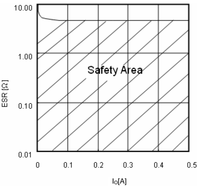
Fig.18 ESR condenser
