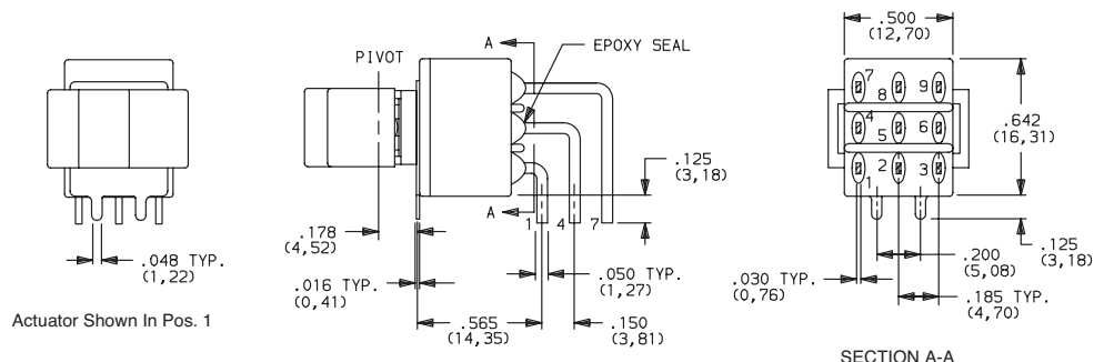
E301J1ABE2 Horizontal Actuation 3PDT
