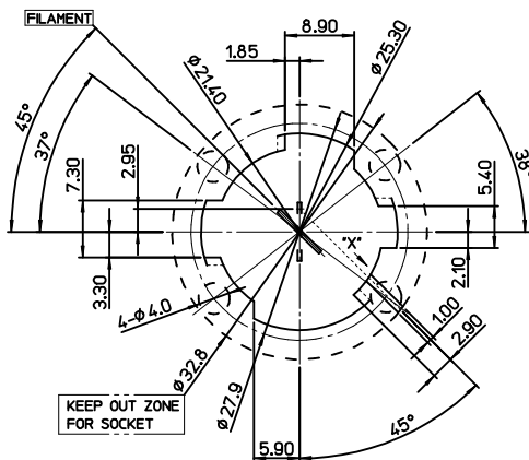
LUG PATTERN "A"
