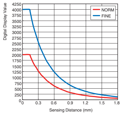
E2CY-X1R5A/E2CY-C1R5A-1
