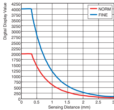
E2CY-C2A(F)
