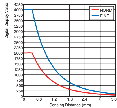
E2CY-V3A
