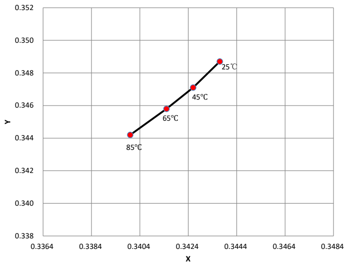
T_j vs. CIE x, y Shift
