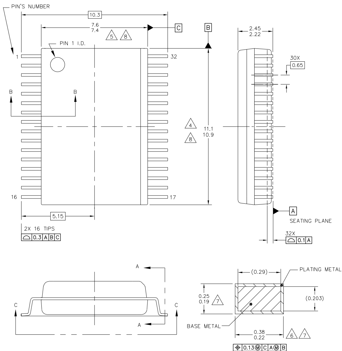
SECTION A-A
