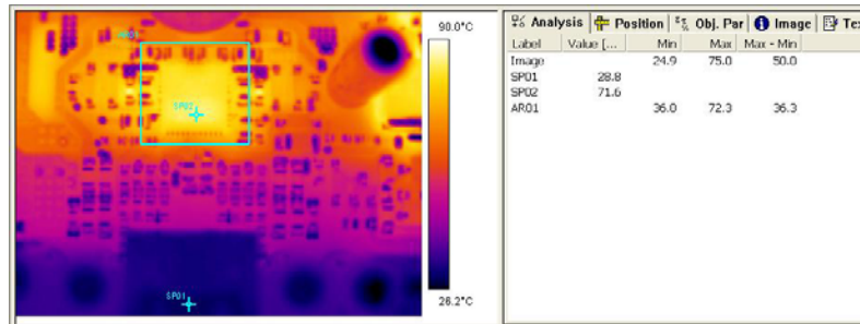
Fig 7 IRAUDAMP18 (Vbus=31V)
