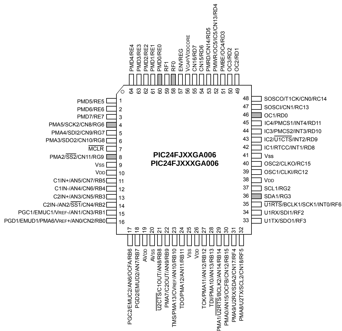
64-Pin TQFP/QFN (1)
