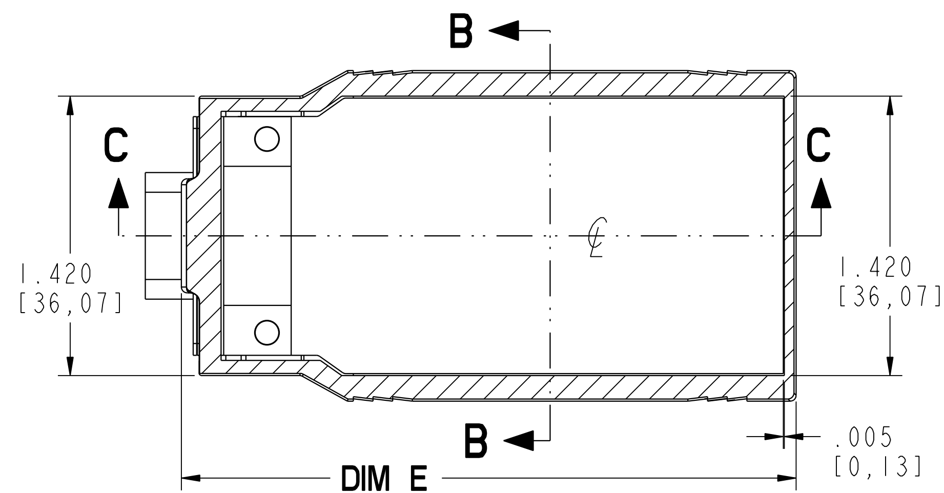
SECTION A-A
