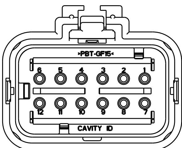
776437-4 SCALE 2:1
