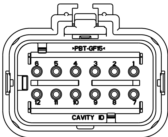
776437-3 SCALE 2:1
