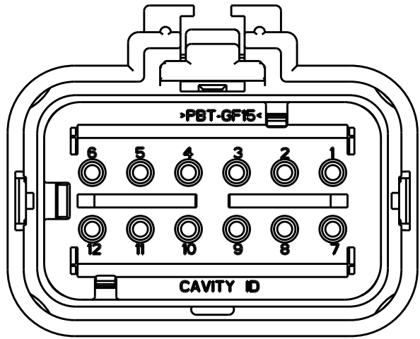
776437-2 SCALE 2:1
