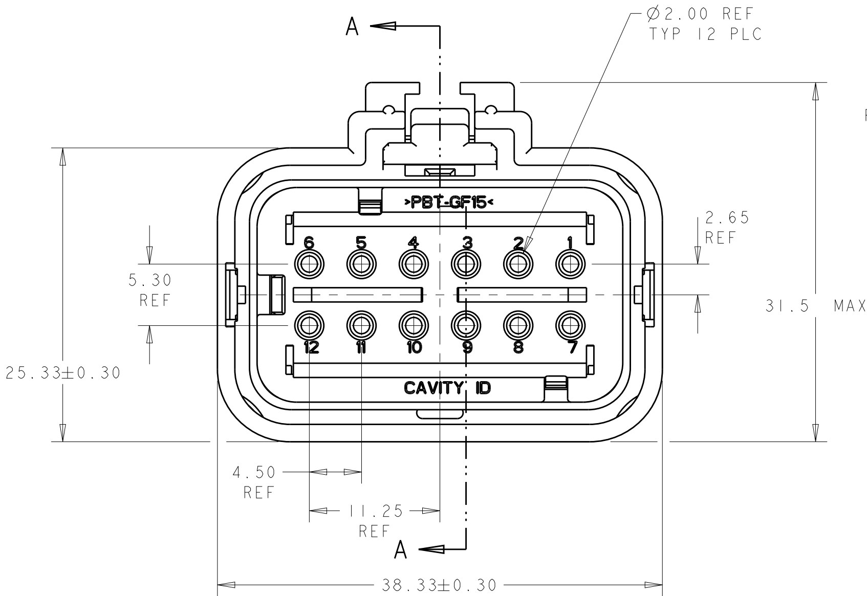
776437-1 SHOWN
