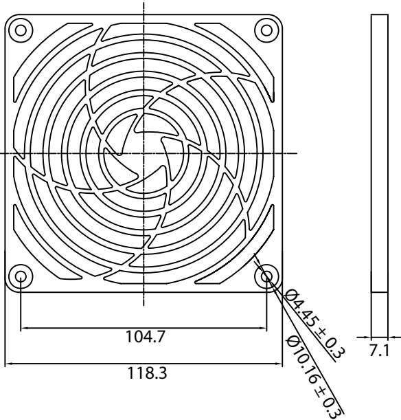
FAN GUARD
