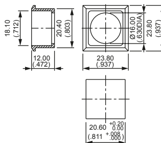
Square : A01FM
