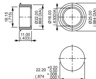
Round : A01FM2
