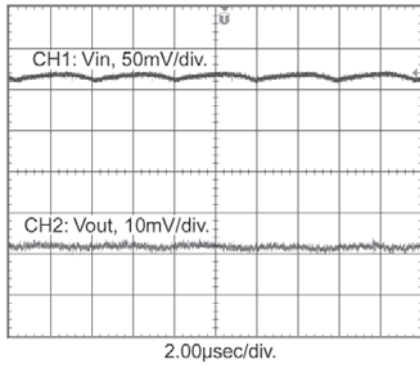
7803SR-C V_{in} = 12\text{V} , I_{LOAD} = 50\text{mA}
