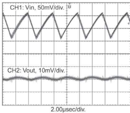
7803SR-C V_{in} = 12\text{V} , I_{LOAD} = 500\text{mA}
