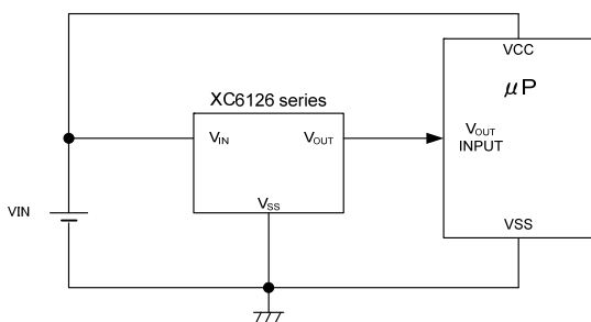
CMOS output
