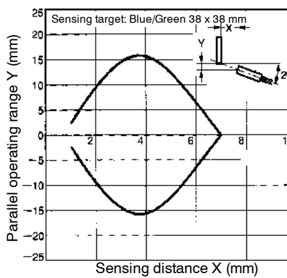
E32-DC200 with E3X-H11 amplifier
