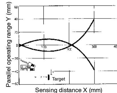
E32-T11L with E39-F3 and E3X-NH amplifier
