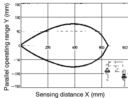
E32-T11L with E39-F1 and E3X-NH amplifier
