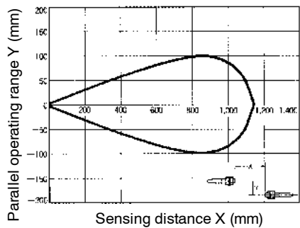
E32-M21 with E3X-NH amplifier
