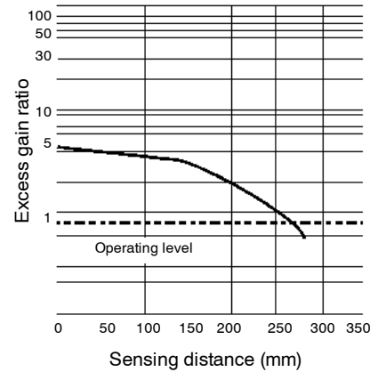
E32-UDBT1-6F with E3JU-X amplifier
