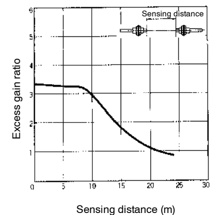
E32-T17L with E3X-NH amplifier
