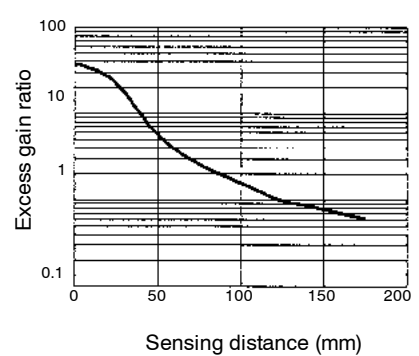
E32-UDBT1-6F with E3JU-X amplifier
