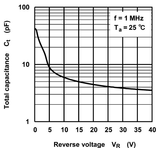
Fig. 8.3 C_t - V_R
