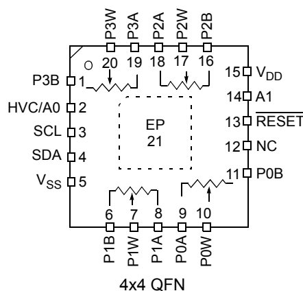
4x4 QFN
