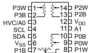
TSSOP
