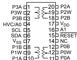
TSSOP
