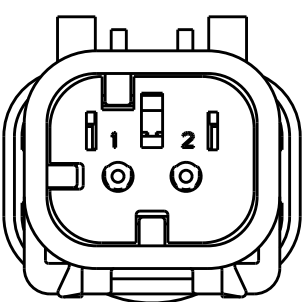
776534-3 SCALE 2:1 KEY C
