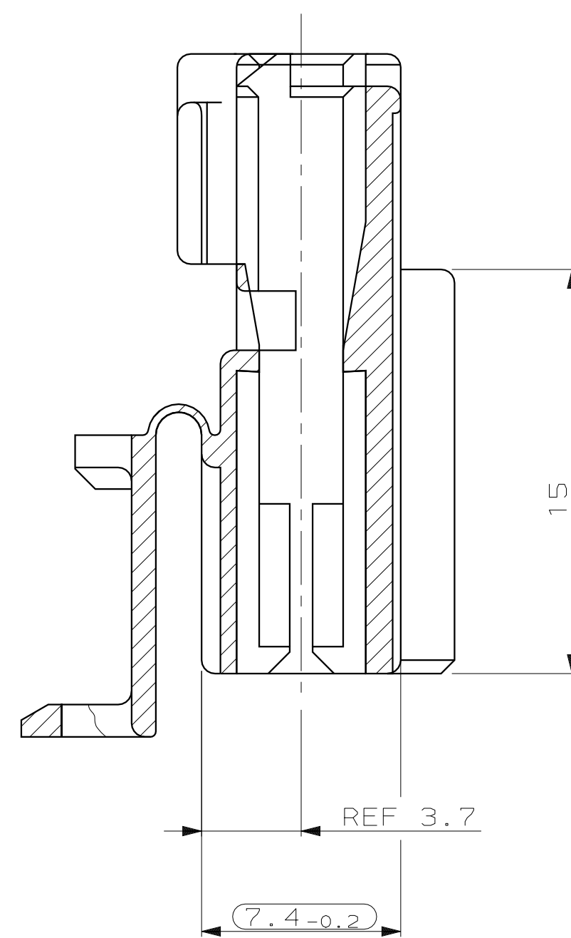
Schnitt A-A
