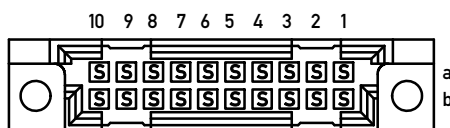
Bestückungsplan / contact layout
