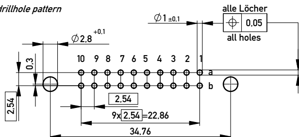
Leiterplatten-Lochbild / PCB drillhole pattern
