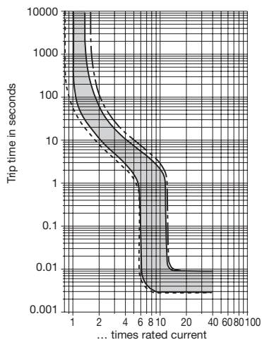
-T1 0.1...6 A
