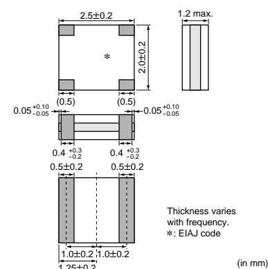
CSACW_X 20.01-70.00MHz
