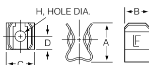
45° Angle Solder Lug Type
