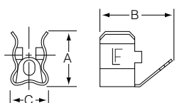
45° Angle Solder Lug Type
