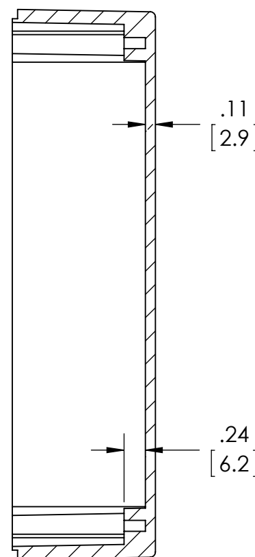
SECTION A-A
